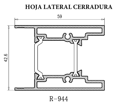
HOJA LATERAL CERRADURA
