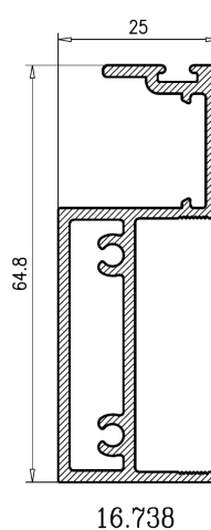
HOJA CIERRE INVERTIDA
