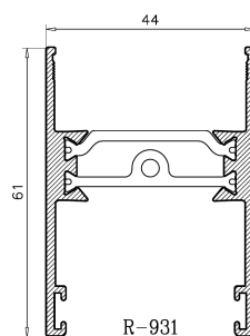
HOJA RODAMIENTO CORREDERA
