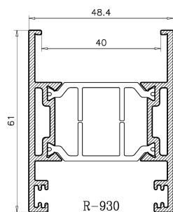
HOJA LATERAL CORREDERA
