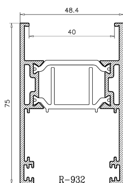
HOJA LATERAL ELEVABLE
