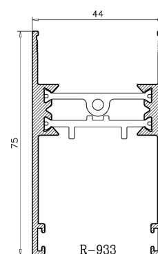
HOJA RODAMIENTO ELEVABLE
