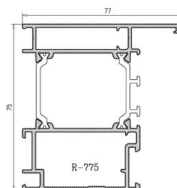
MARCO PUERTA
