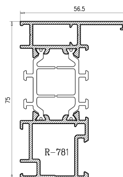
MARCO VENTANA
